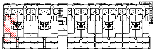
PLANTA PRIMERA
